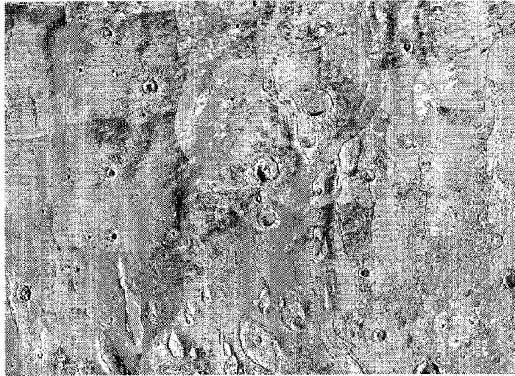
Fig. 2 Tiu Vallis. Image Set image #4.
