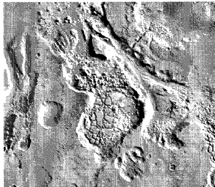
Fig. 3 Hydaspis Chaos, the source of Tiu Vallis.
